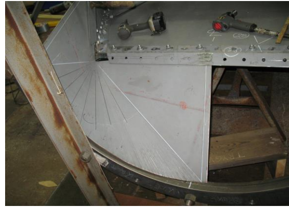
Montering mellom firkant og flens
